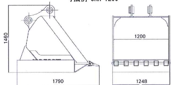
寸法例 SRK-1200
